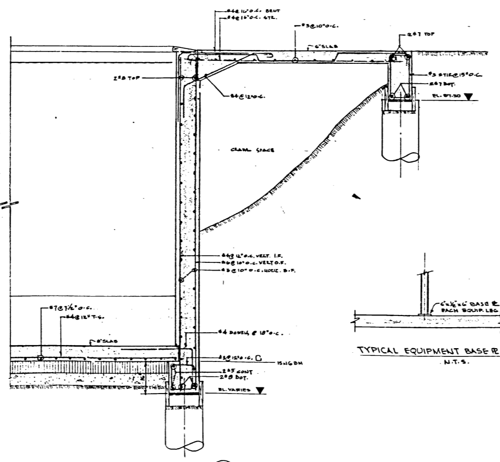
SECTION 3 SCALE: 1/2" = 1'-0"
