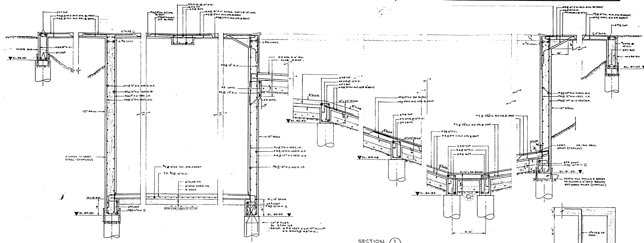
SECTION 1 SCALE: 1/2" = 1'-0"
